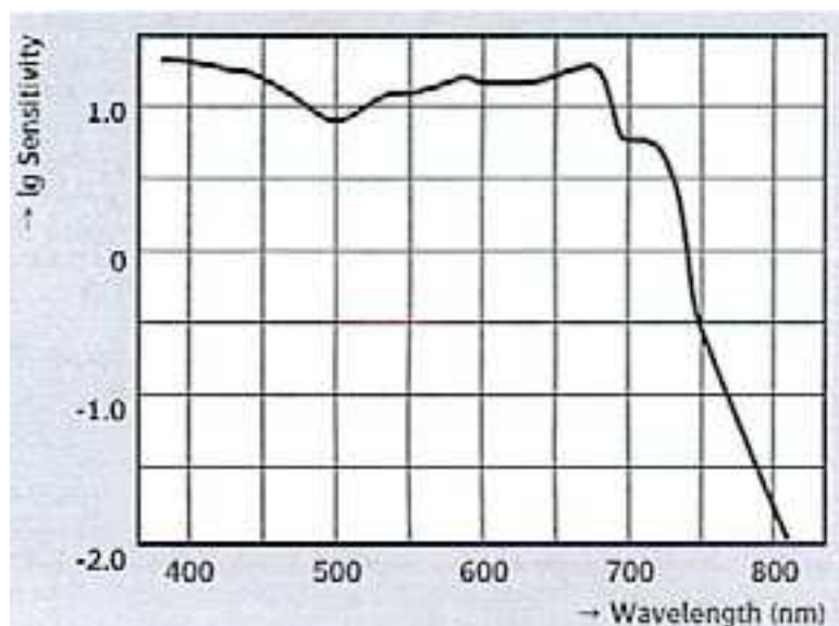
Spektrale Empfindlichkeit
